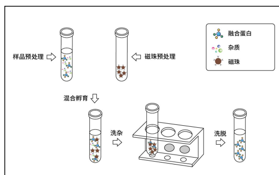
图 1. Magneti-G Myc 标签免疫沉淀/免疫共沉淀试剂盒的使用流程图
