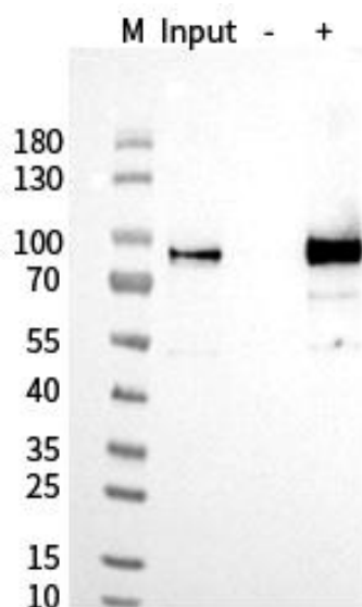
图 2. Magneti-G Myc 标签免疫沉淀/免疫共沉淀试剂盒进行 IP 后的 WB 图
